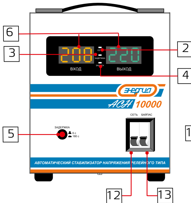
Лицевая панель
