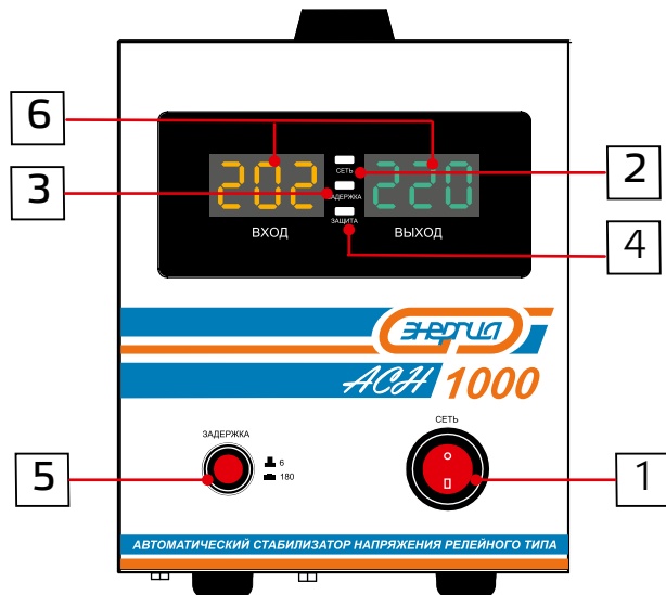
Лицевая панель
