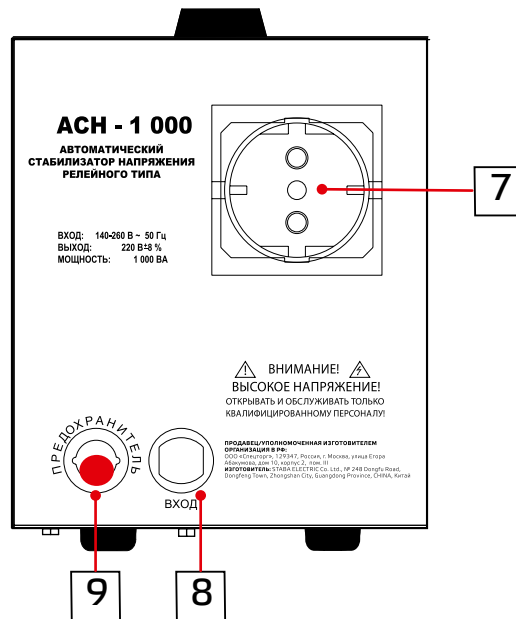
Задняя панель
